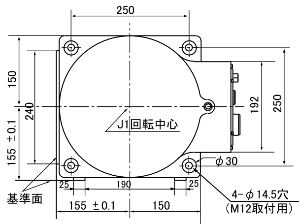
ベース取付寸法(B-B視)
