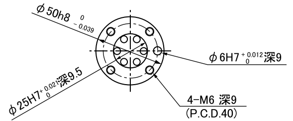
ツール取付面詳細(A視)
