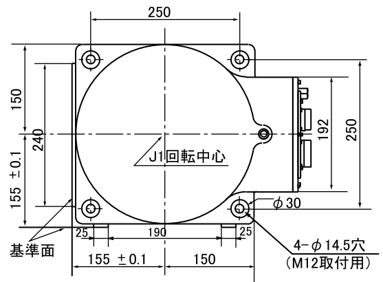
ベース取付寸法(B-B視)
