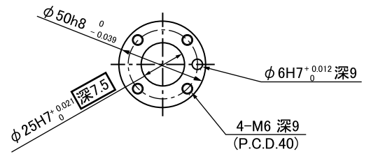
ツール取付面詳細(A視)
