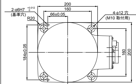
ベース取付面 (上面より)
